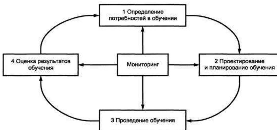
Рисунок 2 - Цикл обучения
